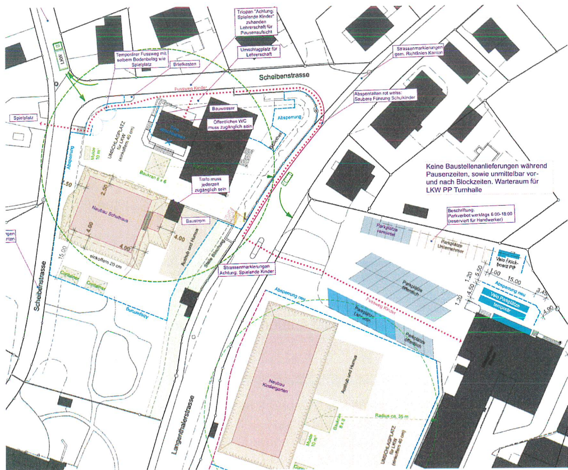
Prov. Baustelleneinrichtungsplan
